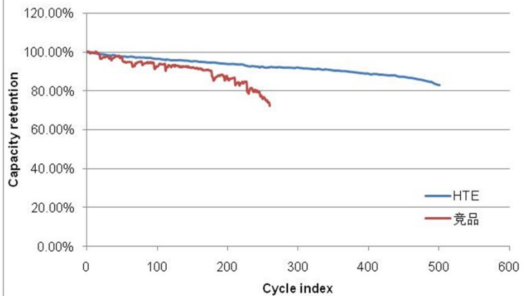
1500 mAh软包圆柱 15A循环性能
