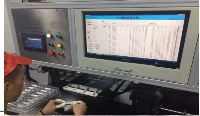
自动OCV测试分选机 Automatic OVC Testing & Sorting Machine
