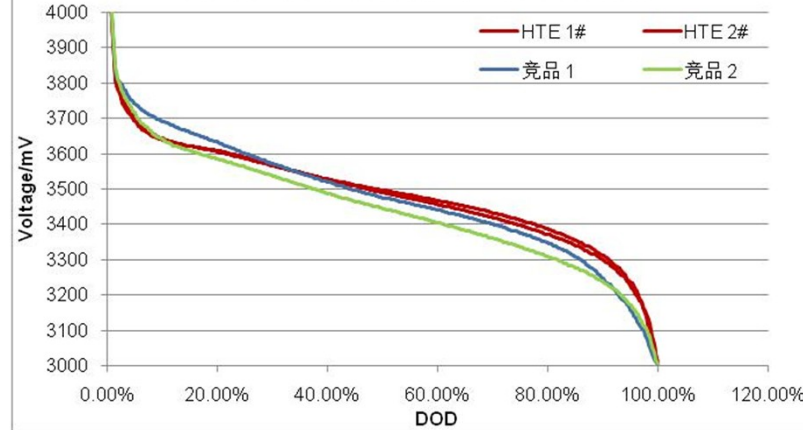
300mAh软包方形 10C放电曲线
